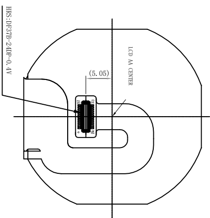
FPC弯折示意图 展开出货
